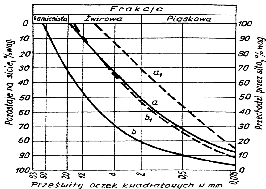
Rysunek 1. Obszar uziarnienia optymalnych mieszank żwirowych
